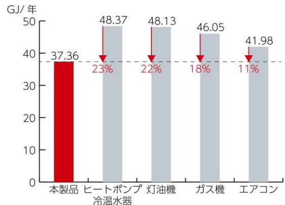
一次エネルギー消費量比較(冷暖房)*1
