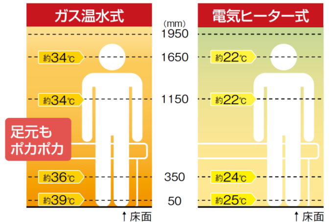
浴室温度分布の比較 (運転開始 15 分後)
