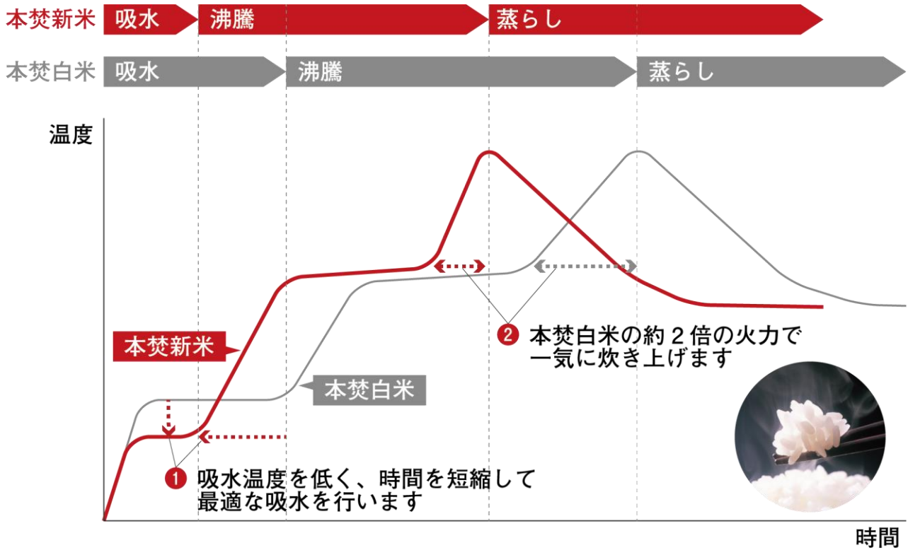
炊飯メニュー別の炊飯釜の温度と時間のイメージ図
